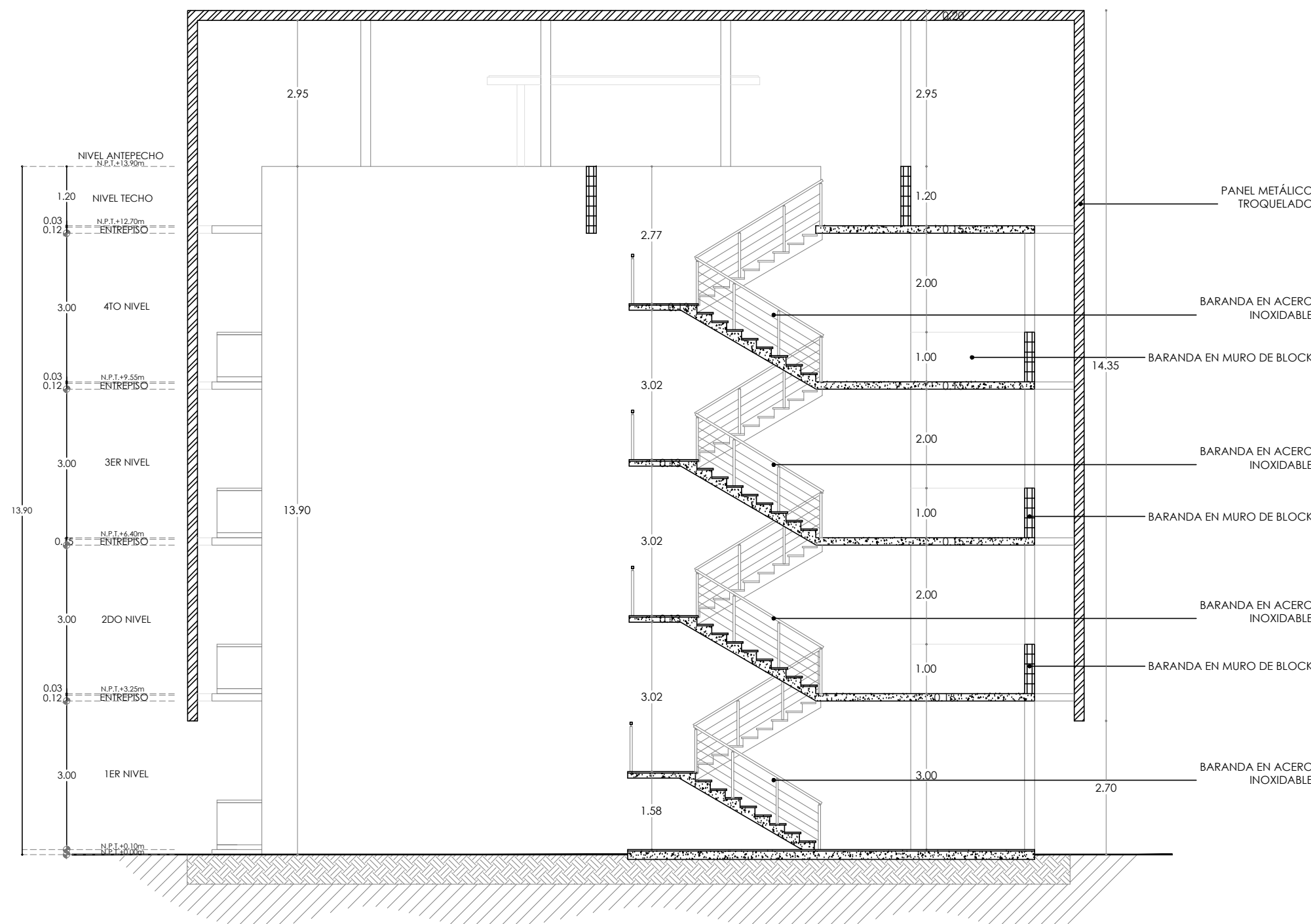
7.1 SECCIÓN A - A' ESC 1:100
