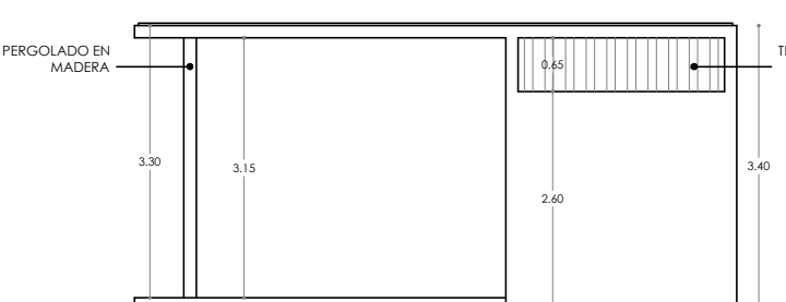
5.7 ELEVACIÓN LATERAL DERECHA ESC 1:100
