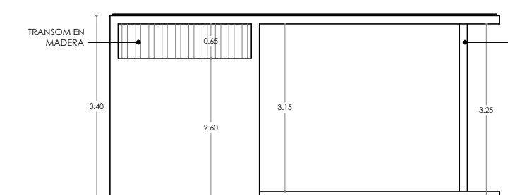
5.9 ELEVACIÓN LATERAL IZQUIERDA ESC 1:100
