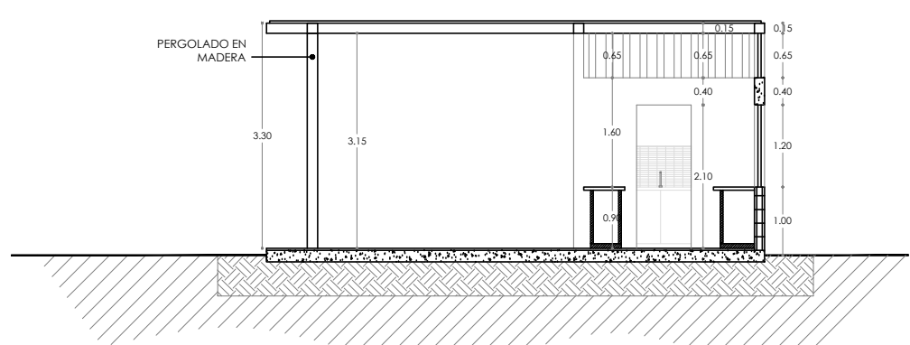
5.10 SECCIÓN A - A' ESC 1:100
