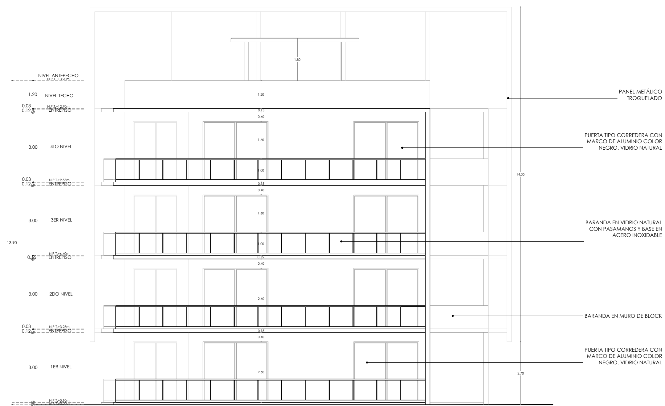
6.2 ELEVACIÓN LATERAL DERECHA ESC 1:100
