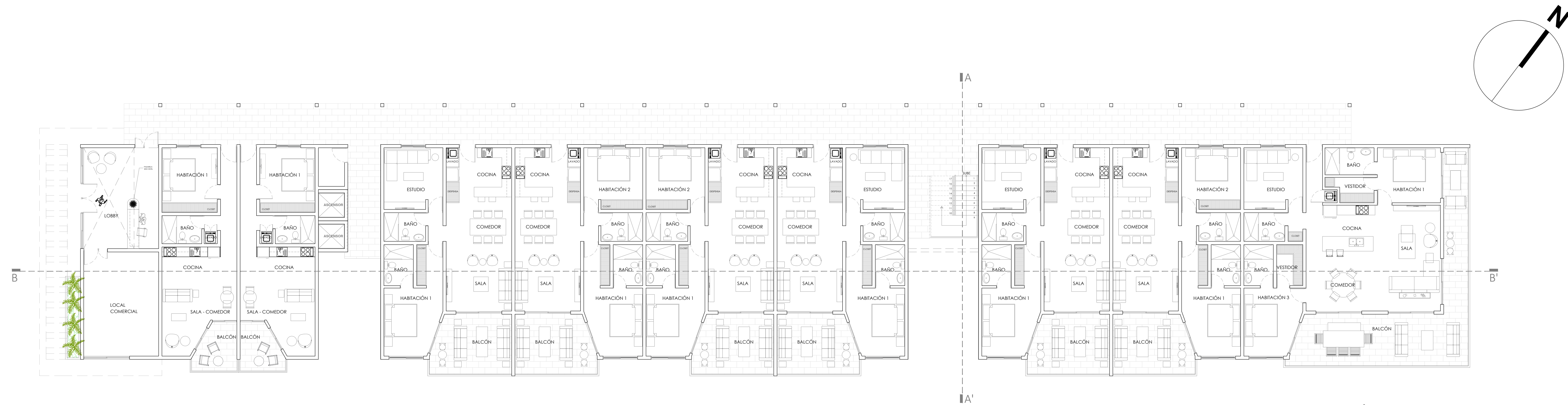
2.1 PLANTA ARQUITECTÓNICA 1ER NIVEL ESC 1:100
