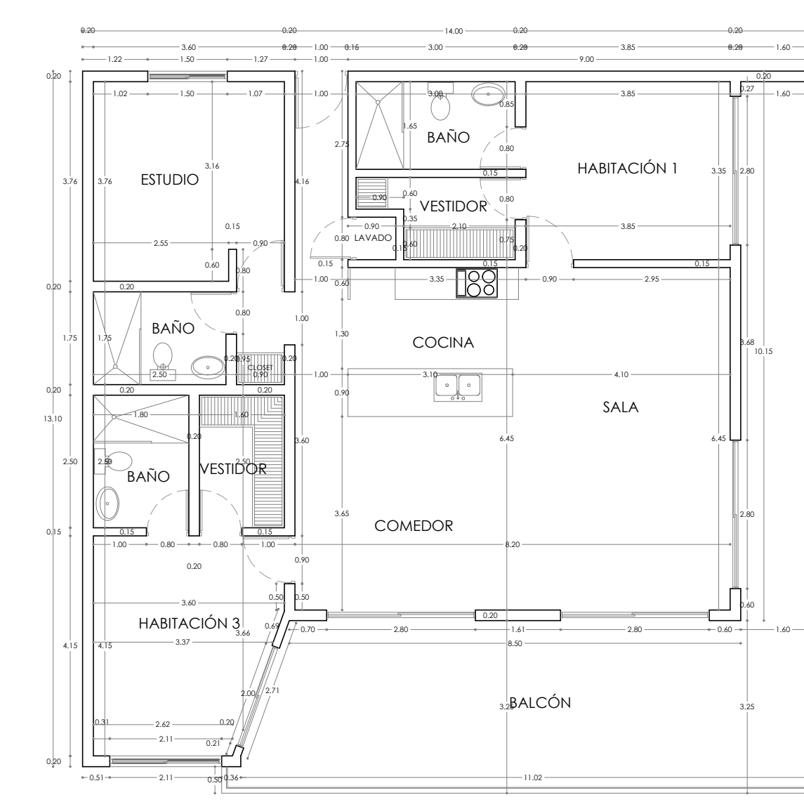
3.3 PLANTAS ARQUITECTÓNICAS TIPO ESC 1:100
