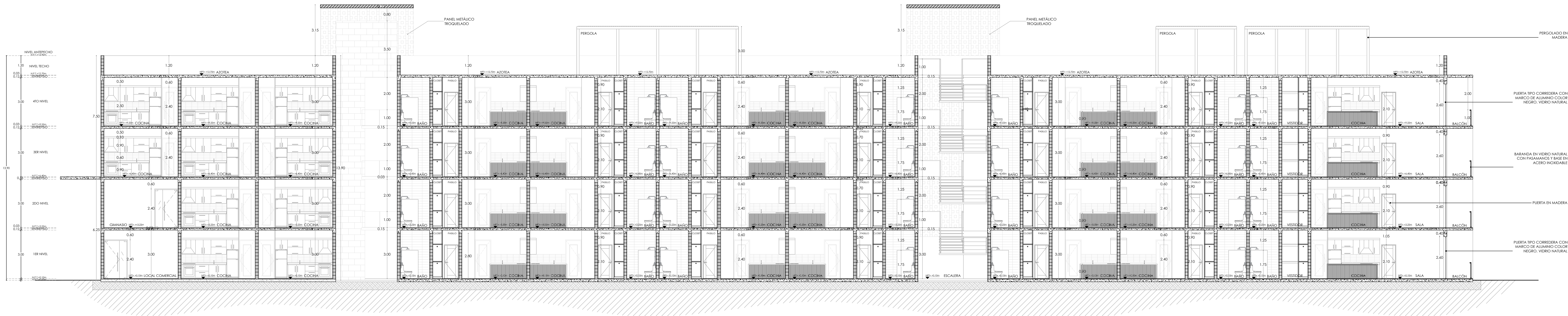
7.2 SECCIÓN B - B' ESC 1:100
