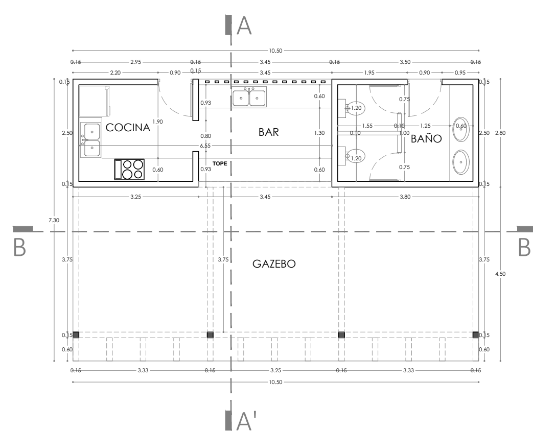
5.5 PLANTA ARQUITECTÓNICA DIMENSIONADA GAZEBO ESC 1:100
