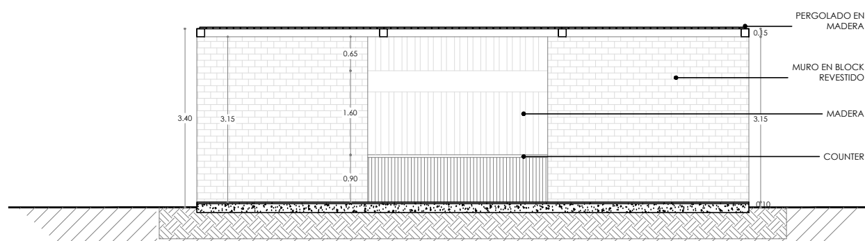
5.11 SECCIÓN B - B' ESC 1:100
