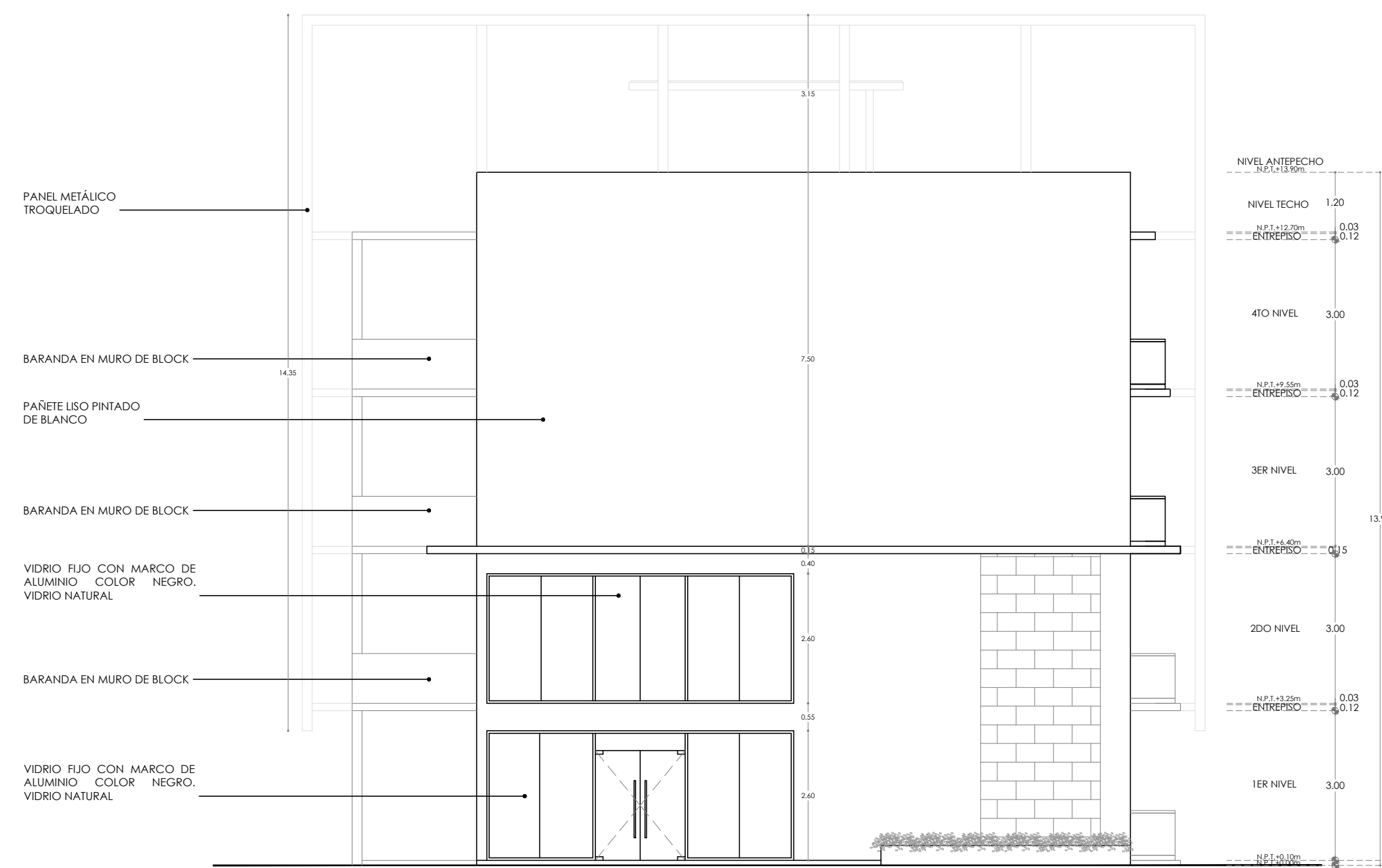
6.3 ELEVACIÓN LATERAL IZQUIERDA ESC 1:100
