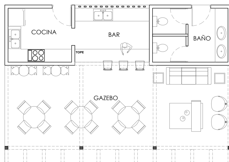
5.4 PLANTA ARQUITECTÓNICA GAZEBO ESC 1:100
